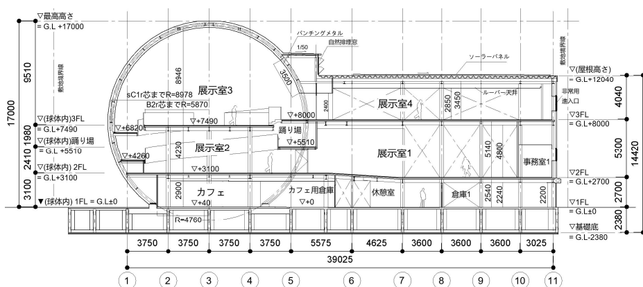
長手方向断面図
