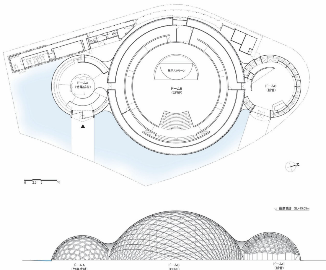
図-1 配置図および断面図
