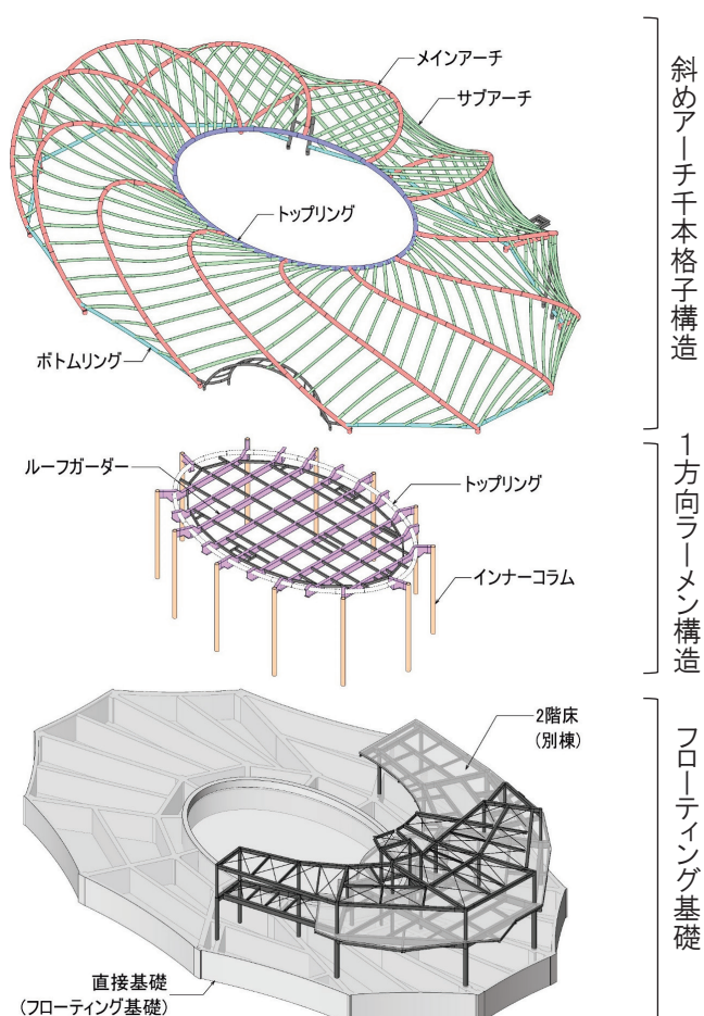
図-1 架構計画
