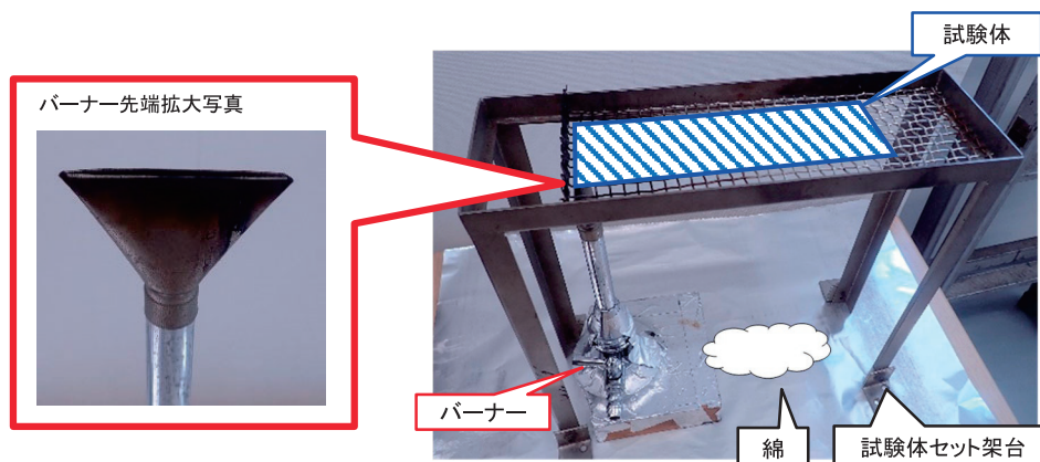
図-1 試験状況のイメージ（燃焼性の等級HF、HBF）
