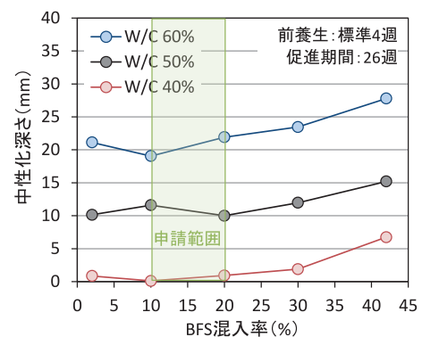
図-1 高炉スラグ微粉末の混入率と中性化深さ
