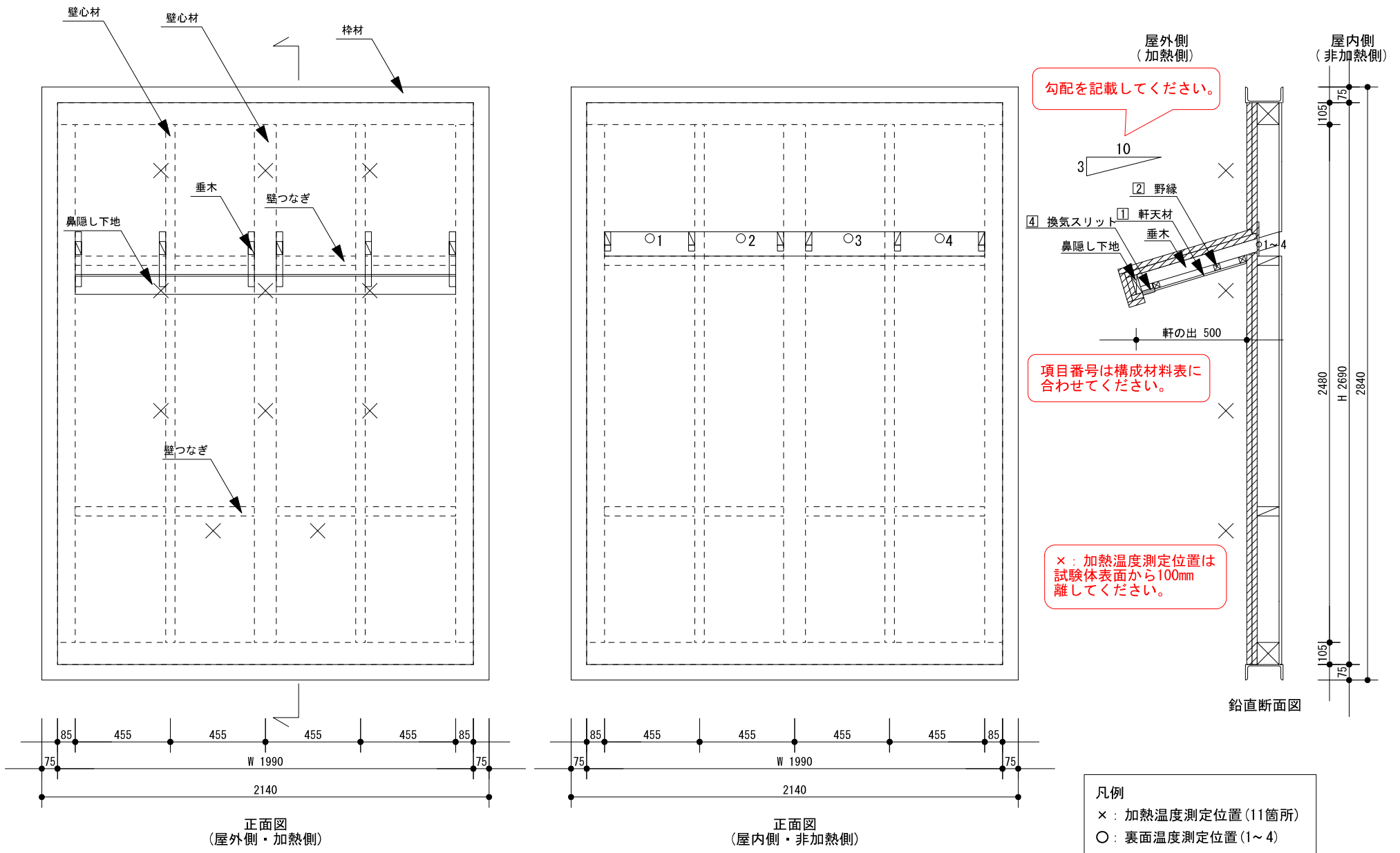
図-1 試験体の構造・寸法・温度測定位置(寸法単位: mm)
