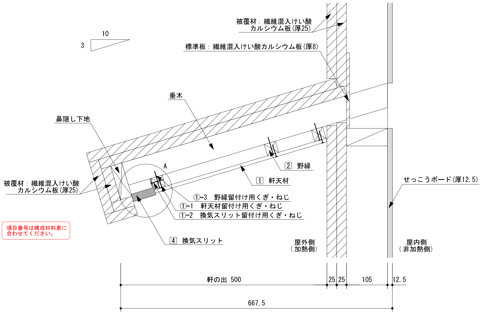
図-2 試験体の構造・寸法 (寸法単位：mm)
