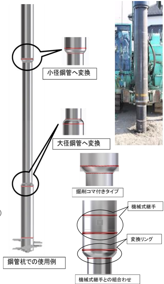
図-1 変換リング工法の使用イメージ
