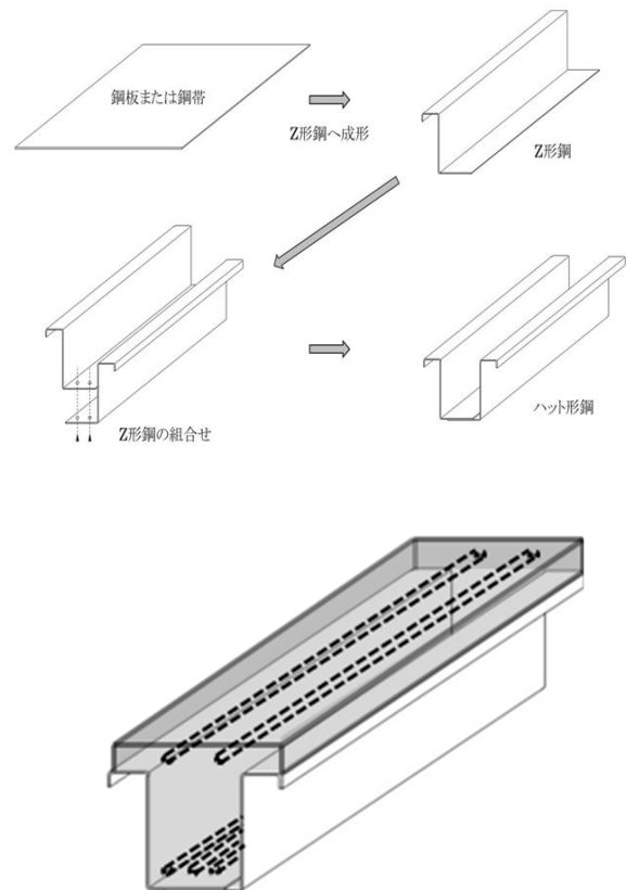
図1 ハット形鋼 SC 梁の概要
