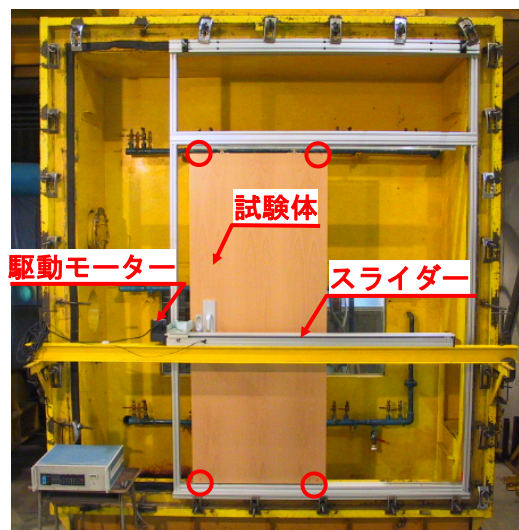
○：戸と枠の隙間を測定
