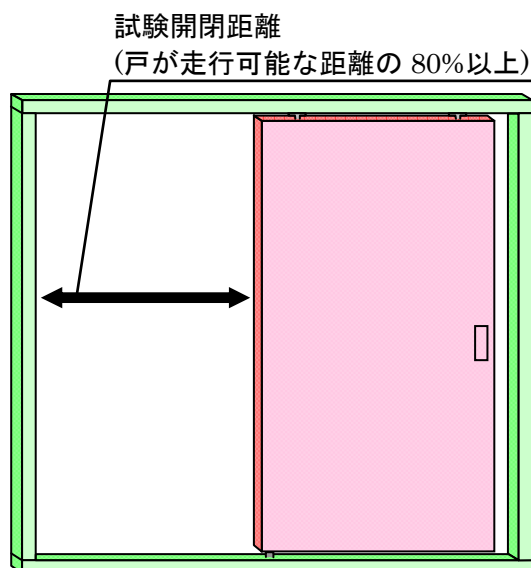
開閉繰り返し試験概要
