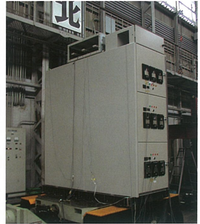
配電盤の耐震実験
