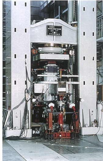
RC造十字形柱梁接合部の実験
