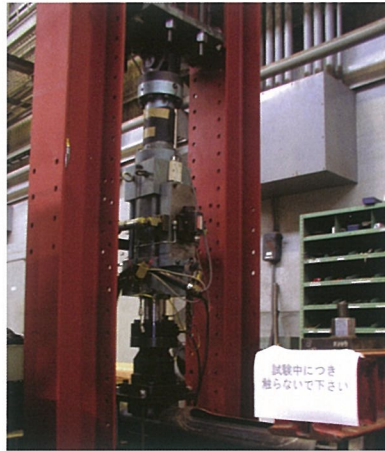
照明灯柱脚部の曲げ疲労実験
