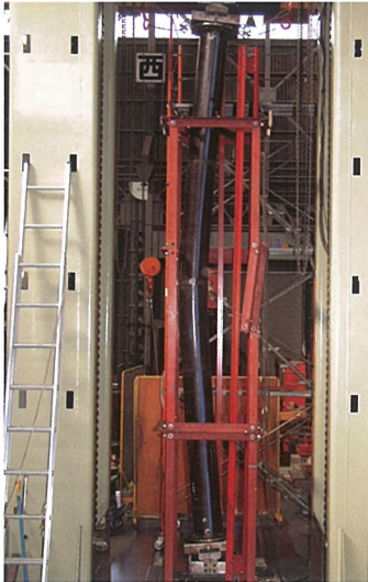
コンクリート充填鋼管の座屈実験
