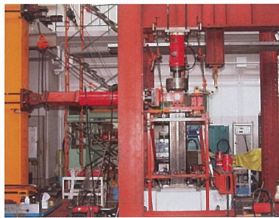
鉄骨露出型柱脚の実験
