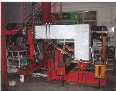
RC造L形部分架構の実験
